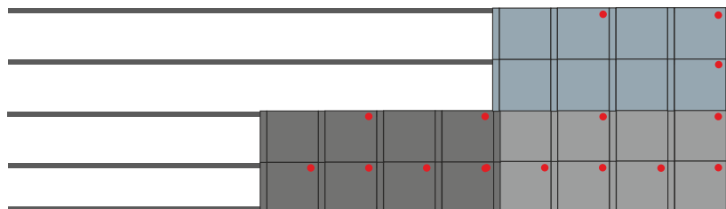
Rys. 9. Schemat rozmieszczenia wkrętów.
